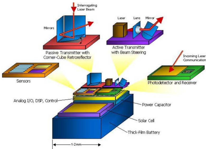
Figur 3.10 Intelligent støv eller "smart dust". Selve støvkornene er store (1 – 2 mm) i nanoteknologiforstand, men sensorelementene, energiforsyningen og andre komponenter har potensial for å kunne utnytte nanoteknologiens framskritt, særlig når det gjelder miniaturisering og materialer med skreddersyde egenskaper.
